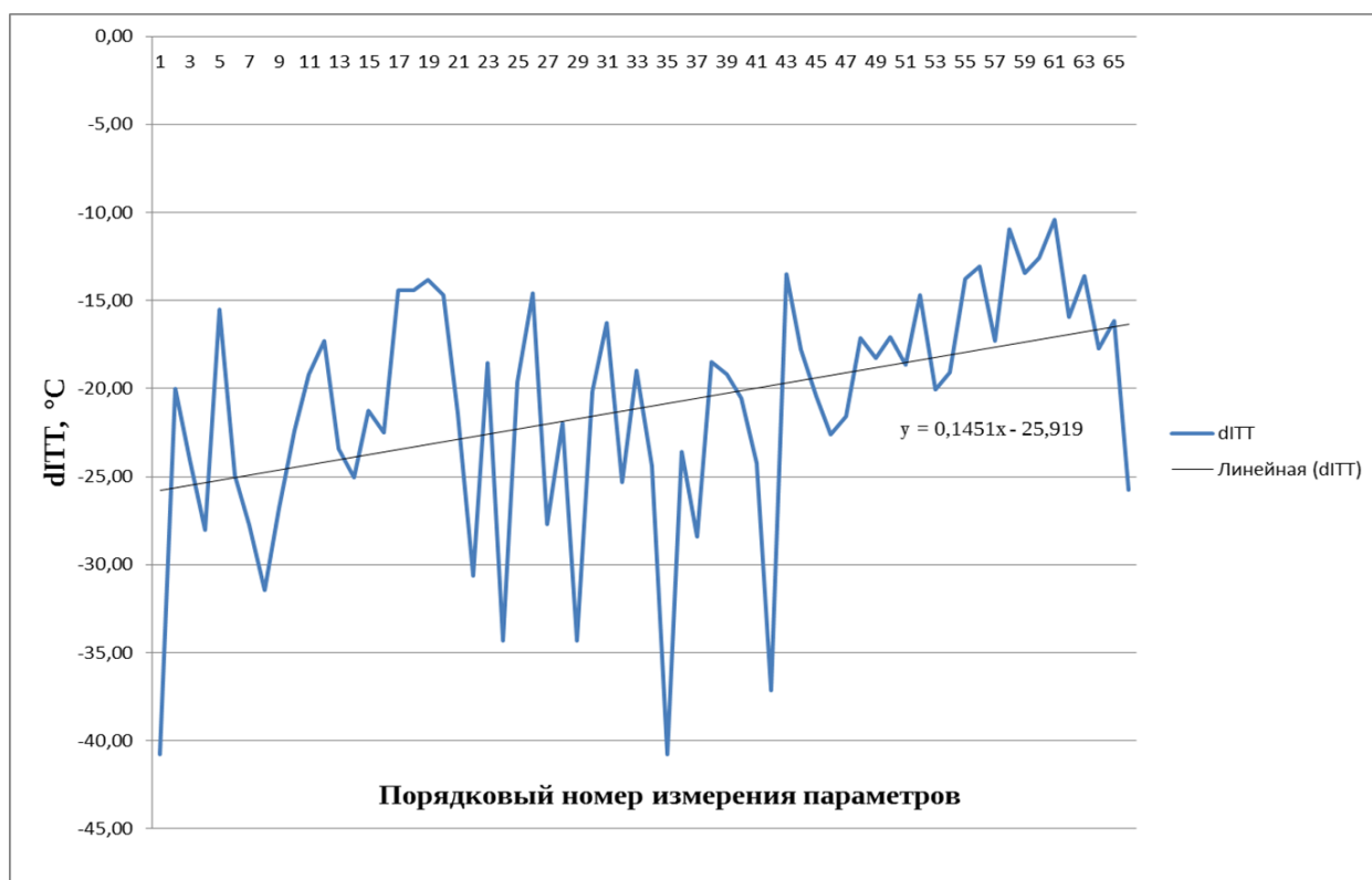
Рисунок 4 – Изменение дифференциальных значений параметра \Delta ITT в ходе измерений
